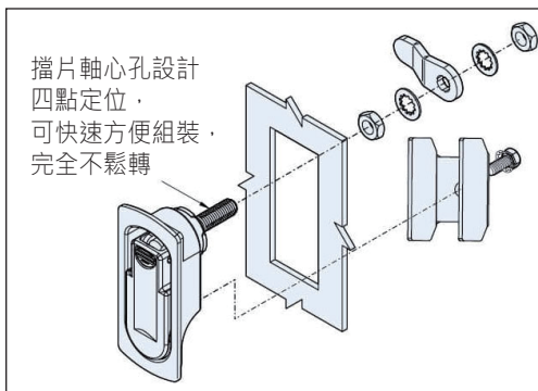
安裝示意圖
