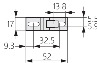
安裝座子尺寸圖
