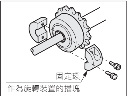
安裝示意圖
