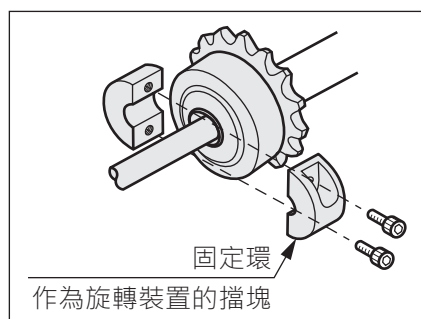
安裝示意圖
