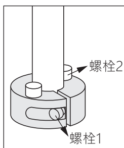
安裝示意圖
