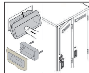
安裝示意圖
