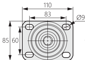
歐式底板尺寸
