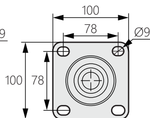
日式底板尺寸
