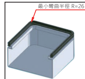
安裝示意圖
