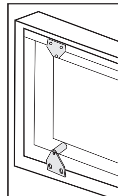
安裝示意圖
