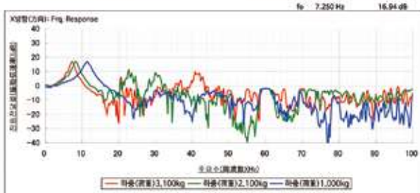
Q-INTOP 마운트「SR160」평가시험(マウント「SR160」評価試験) 중량(重量): 1,000~3,100kg 측정조건(測定条件): 허용하중(許容荷重)800kg / 개(個)
