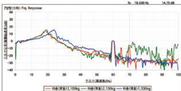
진동전달특성도(振動伝達特性図)(데미-하중상/평상)(ダミー荷重上/床上)
