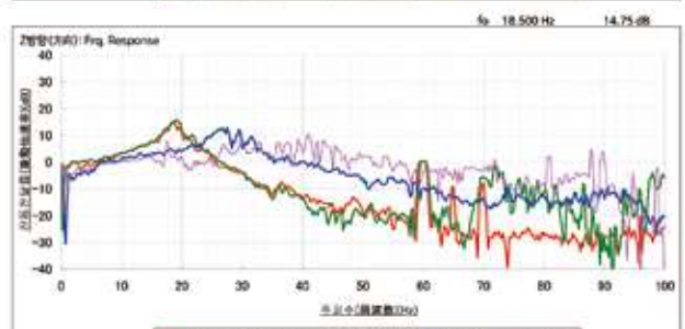
진동전달특성도(振動伝達特性図)(데미-하중상/평상)(ダミー荷重上/床上)
