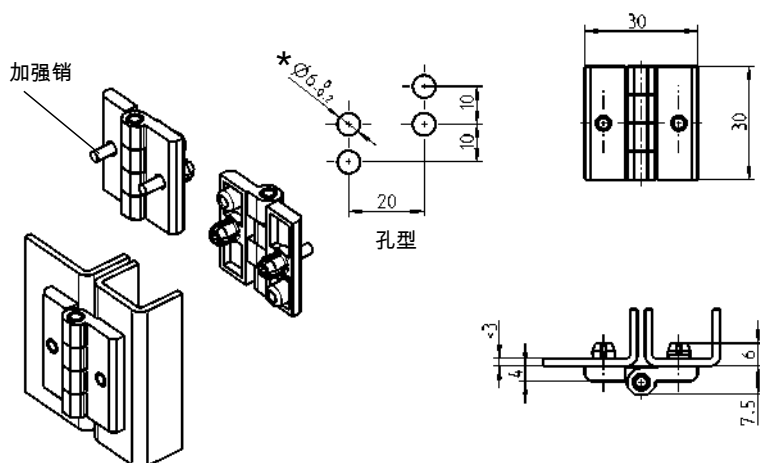
黑色PA铰链、铰链销轴和加强销
