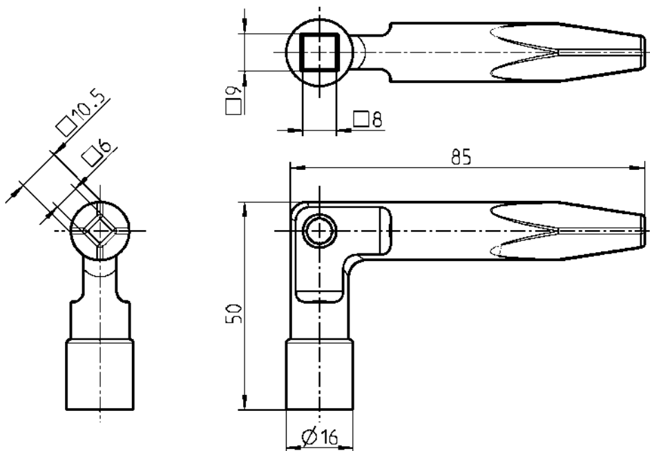
黑色锌合金I型钥匙, 联邦铁路专用
