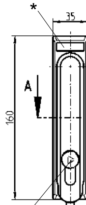
锁定件
