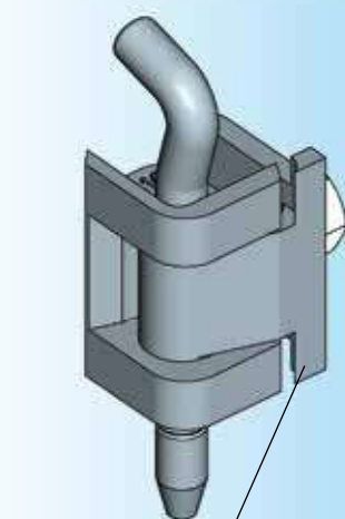
带M6螺纹和销轴的铰链座
