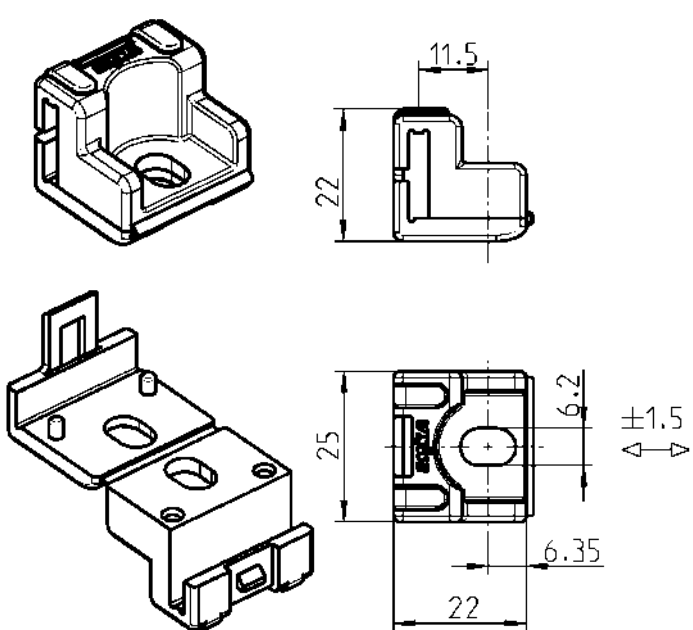
导向件预先安装在连杆上!
