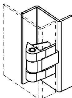
孔型
