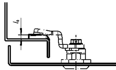
安装示例：显示门和框体内部
