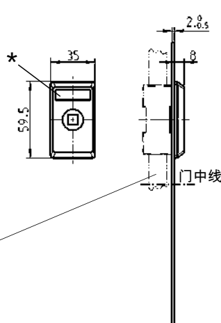
连杆锁
