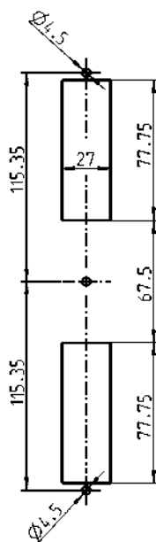
孔型
