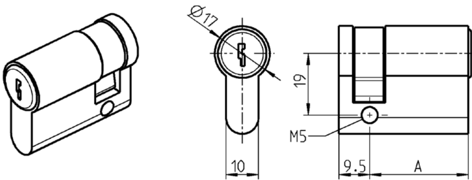
异型半圆柱锁芯和双异型半圆柱锁芯旋转手柄 用于A=30和A=35的异型半圆柱锁芯
