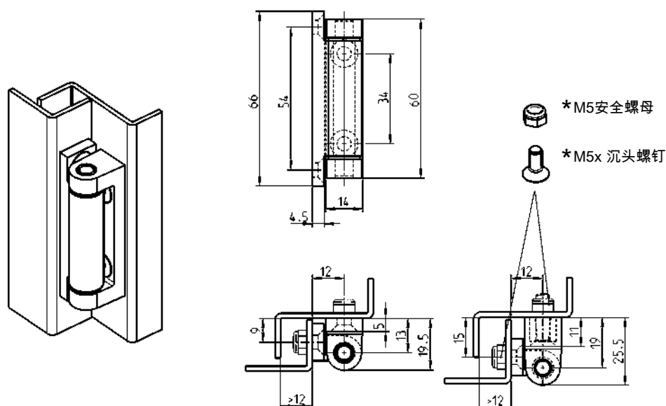
锌合金铰链，不锈钢销轴和PA衬套
