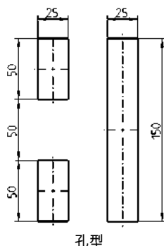
孔型
