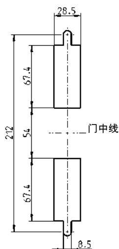
孔型
