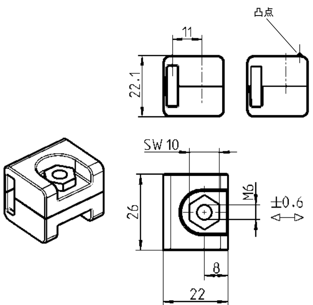
凸点可以避免门与框碰撞发出响声
