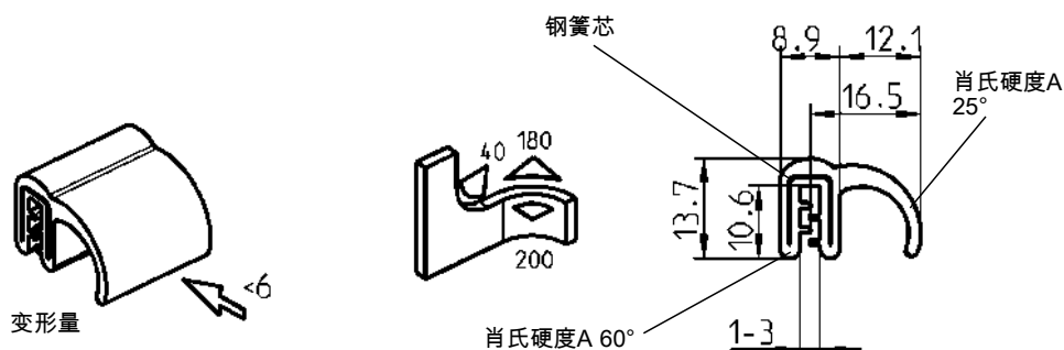
黑色(EPDM)发泡密封胶条, 肖氏硬度A 25°(EPDM夹紧部分, 肖氏硬度A 60°±5)
