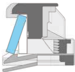
1. 扁连杆卡入到导向件中
