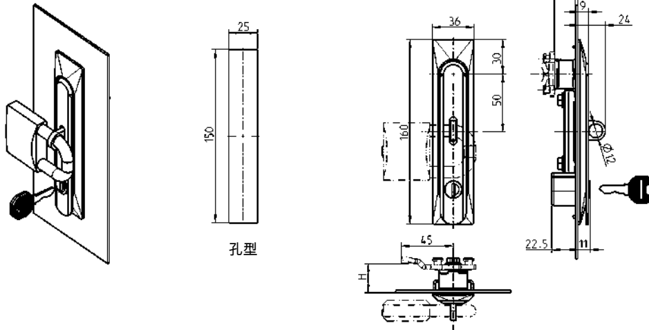
B型带挂锁孔
