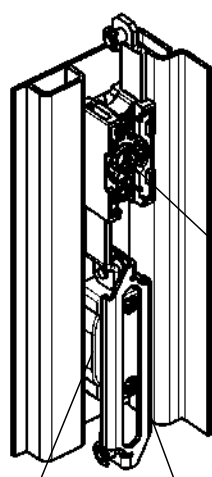
后盖
