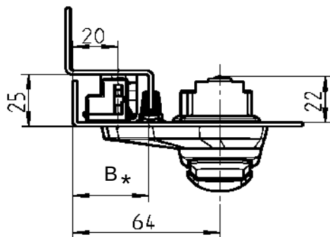
安装示例
