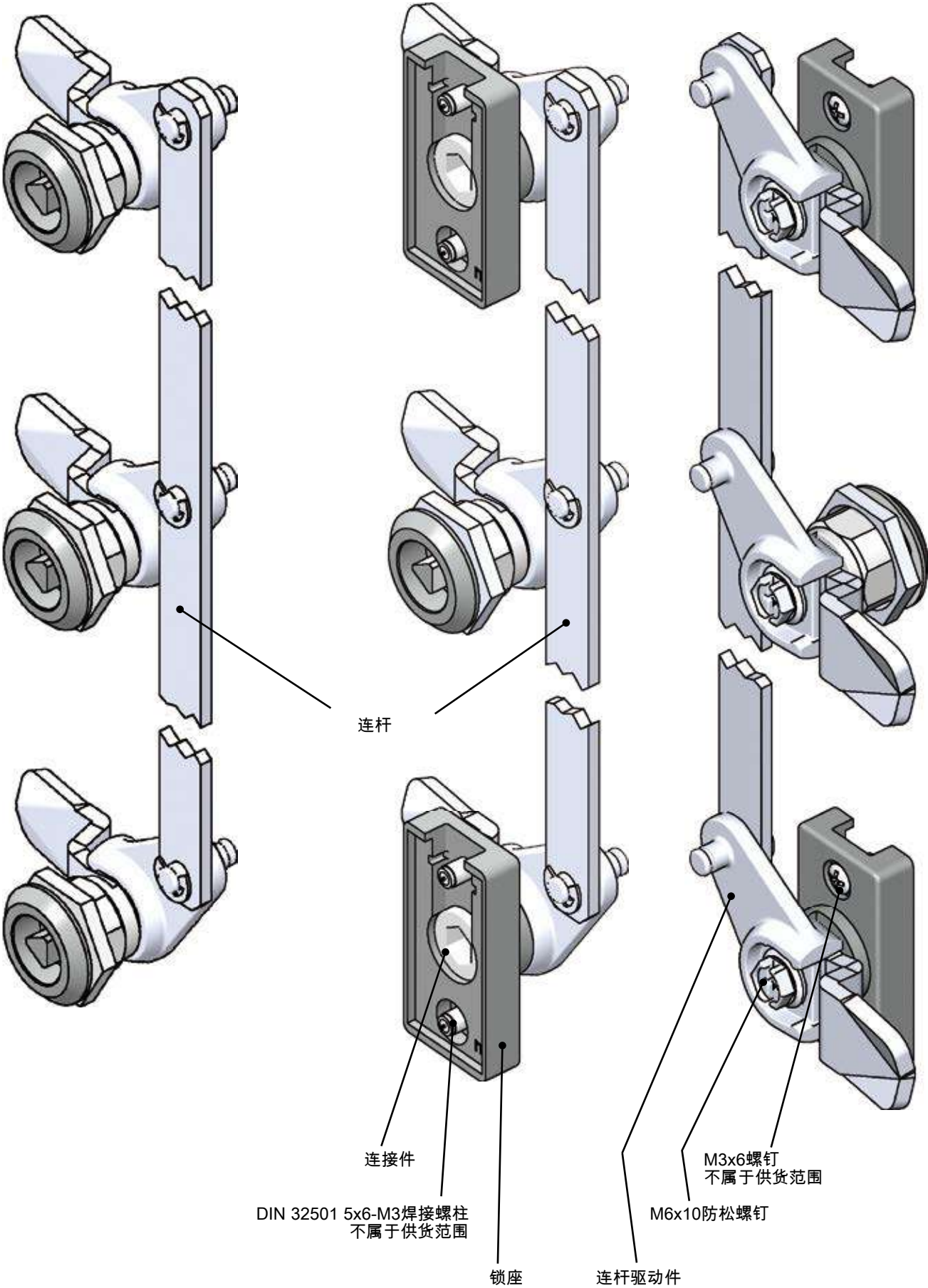
三个转舌锁示例
