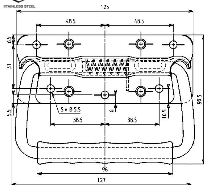
带螺旋弹簧和垫板示意图
