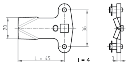
*3型 锁舌及连杆驱动件
