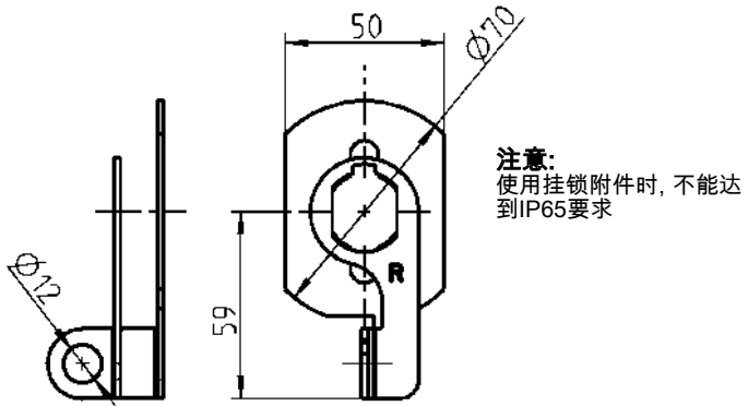
黑色涂层钢挂锁附件
