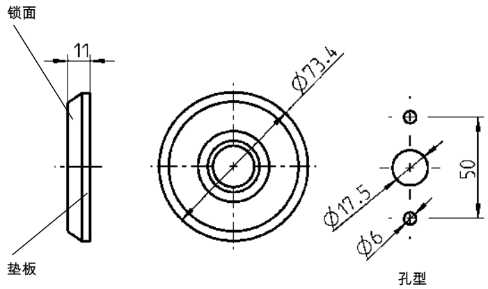
黑色PA+GF锁面
