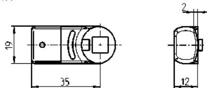
*3型 锁舌及连杆驱动件
