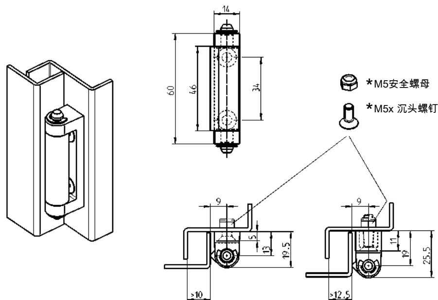
锌合金铰链，裸面钢中间件，镀锌钢销轴和垫圈
