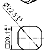
孔型
