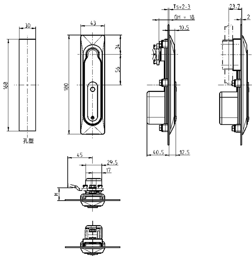
90°锁闭 带锁舌
