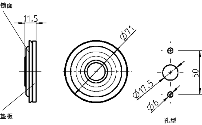
镀锌钢锁面
