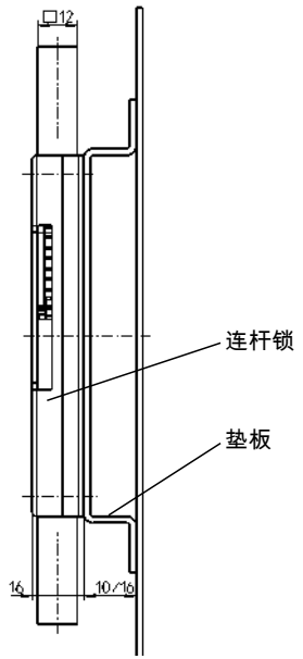
180°锁闭 行程32mm
