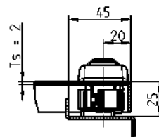
折边空间
