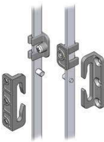
锁闭方式和锁定件
