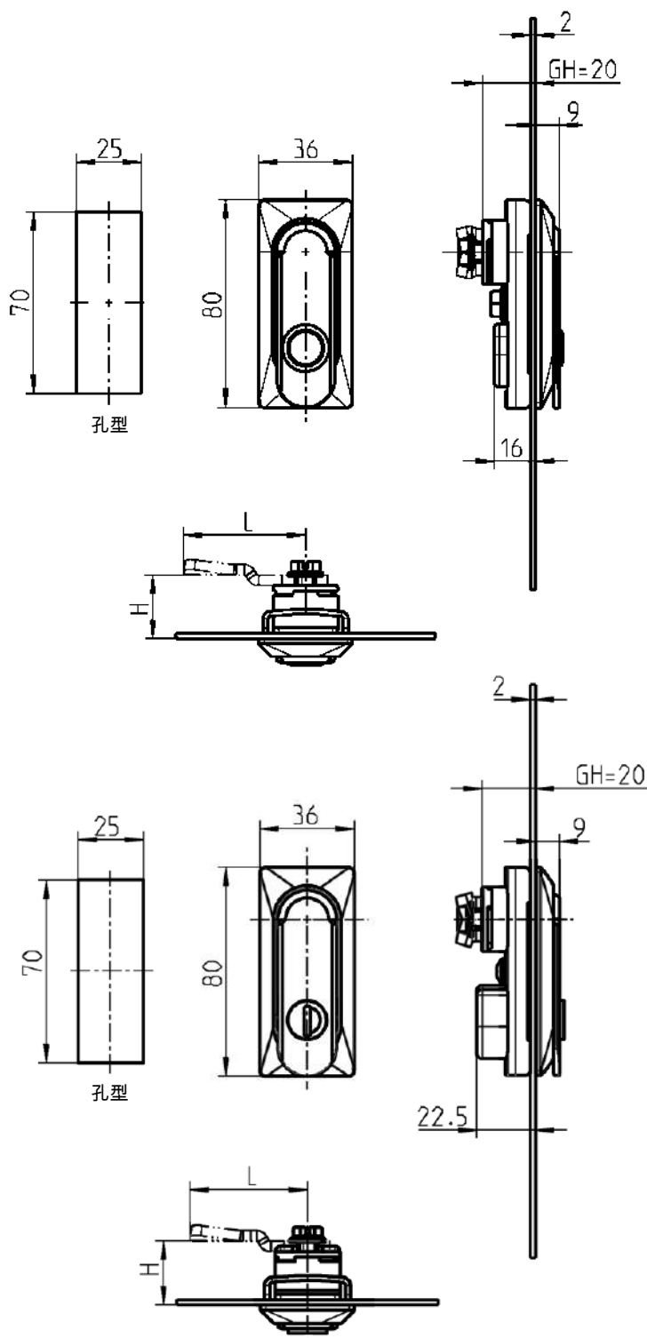
90°锁闭
