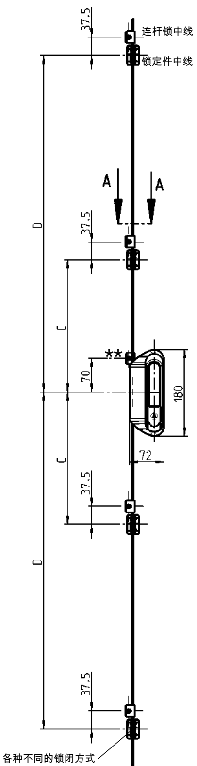
无门显示示例
