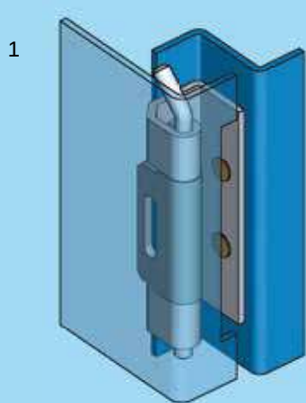
柜门为透明显示
