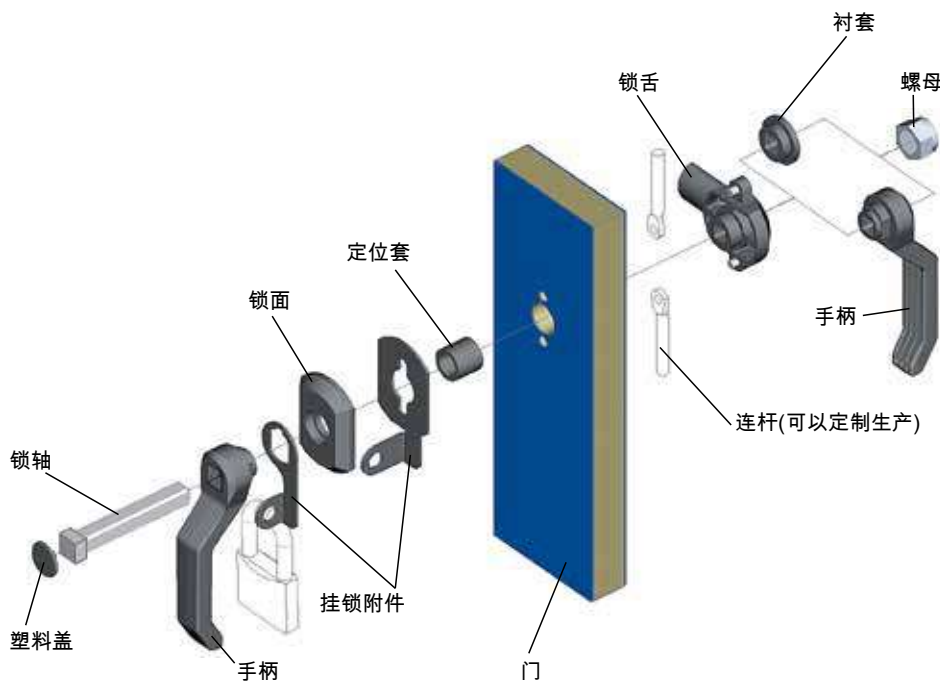
组装示例
