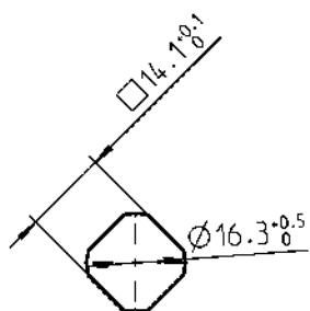
螺母固定或卡式固定孔型
