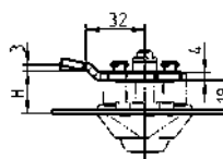
A型: 带T型螺柱锁舌
