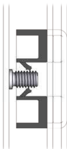
导向件预先安装在连杆上
