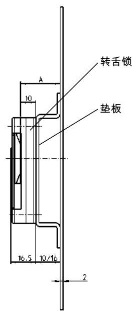
180°锁闭 行程32mm
