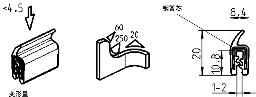
黑色EPDM密封胶条, 肖氏硬度A 60°±5 1011-31
