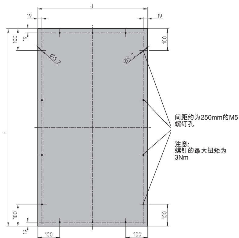
有框铝合金窗的安装尺寸图
