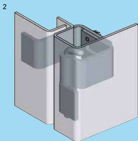
铰链安装透视图
