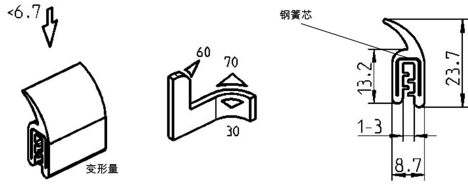
黑色EPDM密封胶条, 肖氏硬度A 60°±5 1011-29
