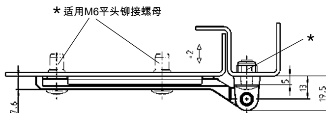
3D螺母固定铰链
