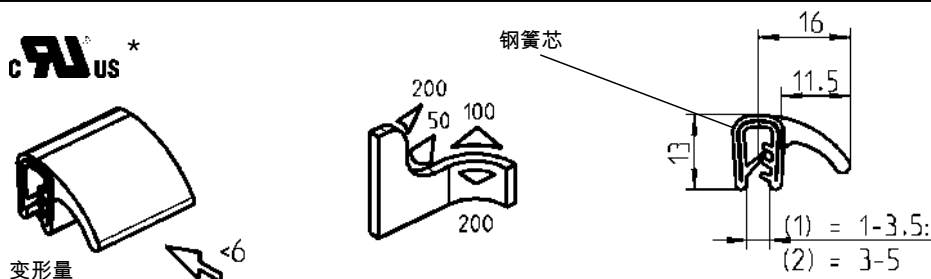
黑色(EPDM)发泡密封条(夹紧部分PVC, 肖氏硬度A 70°±5)
