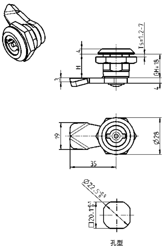
螺母固定
