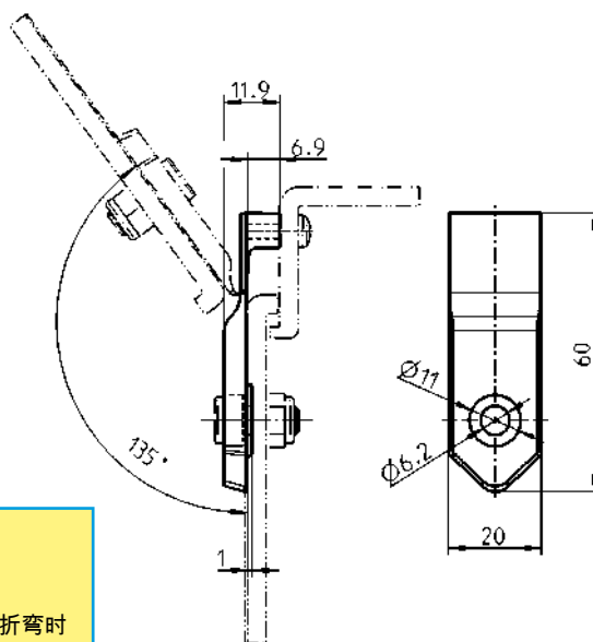
详图A 开启状态
