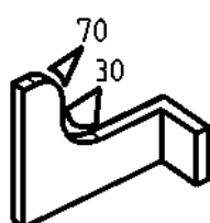
深灰色PVC棱边保护条，肖氏硬度 A 70° ± 5
