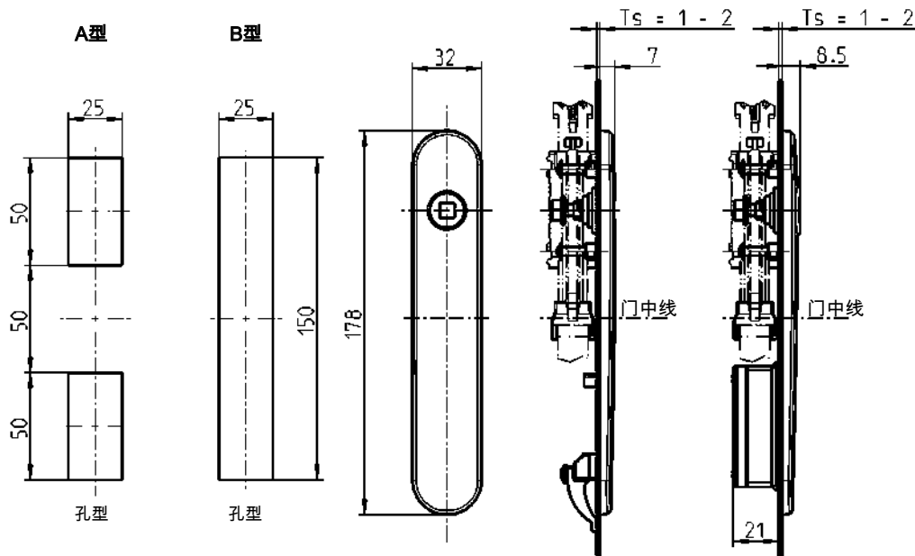
组装示例
