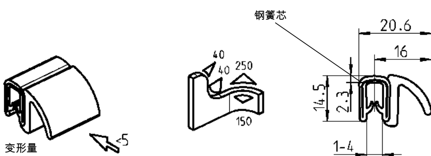
黑色(EPDM)发泡密封条(夹紧部分PVC, 肖氏硬度A 70°±5)
