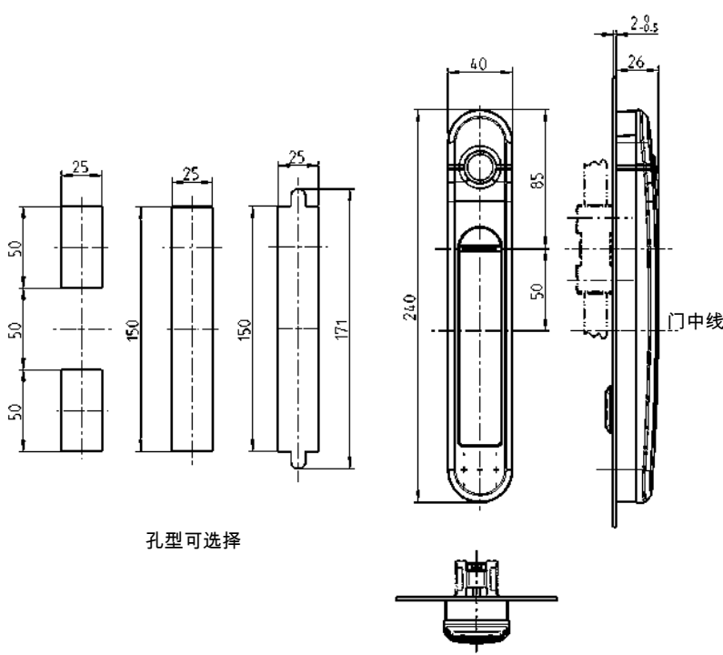
带连杆锁或锁座的旋转手柄
