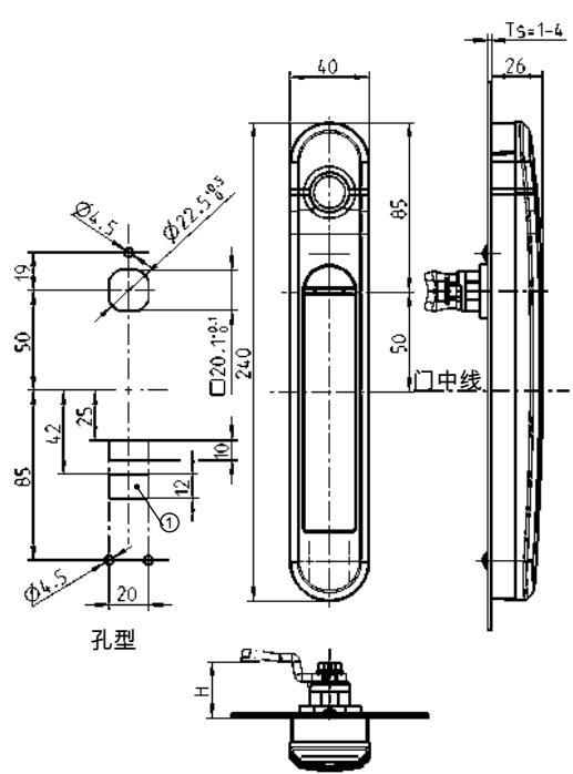
带锁舌的旋转手柄
