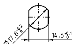
适用于弹簧固定安装的孔型
