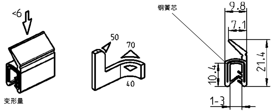
黑色(EPDM)发泡密封胶条(EPDM夹紧条, 肖氏硬度A 60°±5) 1011-37
