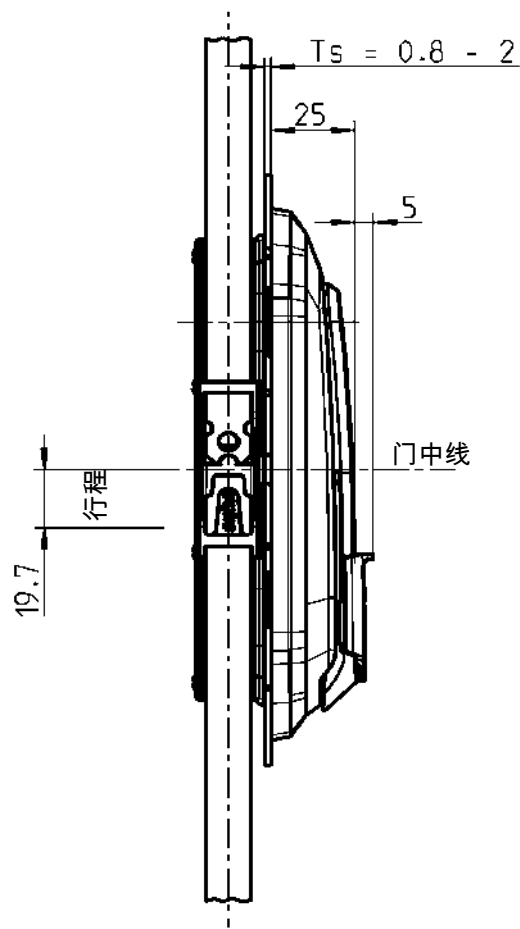
连杆单向行程
