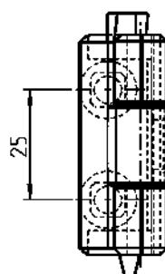
铰链为透明显示
