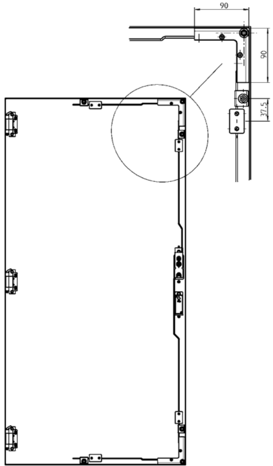
门内安装示例
