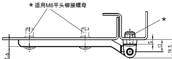
2D螺母固定铰链
