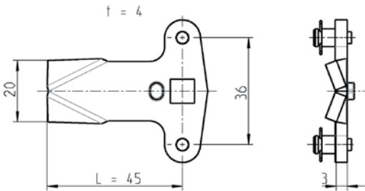
2型 锁舌及驱动件 ( 三点锁舌 )
