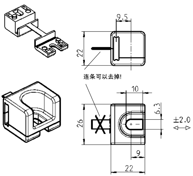
导向件预先安装在连杆上!
