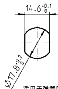
适用于弹簧固定安装的孔型
