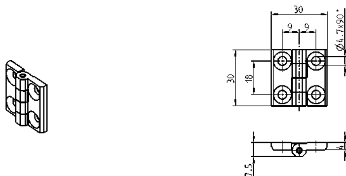
螺钉固定铰链 M4沉头螺钉，锌合金材质，表面处理可选择，不锈钢销轴
