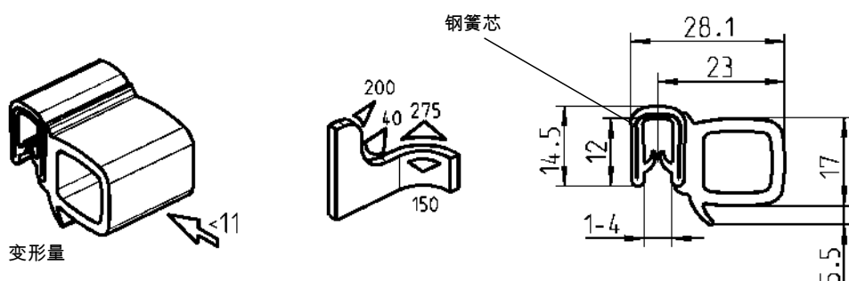
黑色(EPDM)发泡密封条(夹紧部分PVC, 肖氏硬度A 70°±5)
