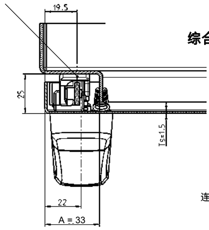
示例 锁闭方式 2
