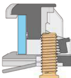
2. 导向件安装在焊接螺柱上
