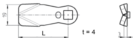
2型 锁舌
