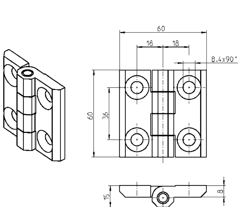
316不锈钢270°螺钉固定铰链，带M6沉头螺钉 (2D螺母)
