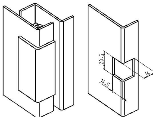
孔型
