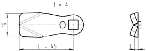
2型 锁舌及驱动件 ( 三点锁舌 )
