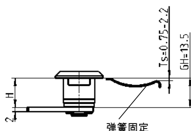
适用于弹簧固定安装的孔型
