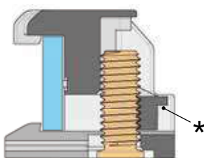
3. 导向件安装完成
