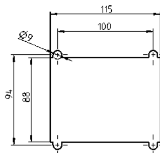
孔型
