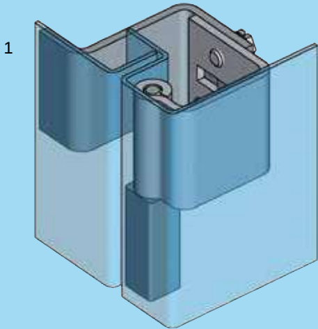
门和柜体为透明表示
