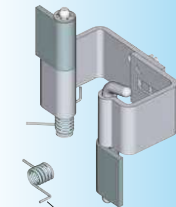
左装式铰链弹簧
