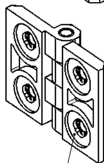
常用的内嵌式M6铆接螺母
