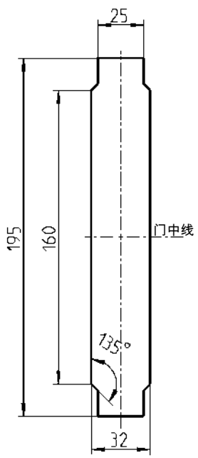
可选孔型
