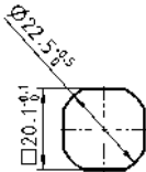
孔型
