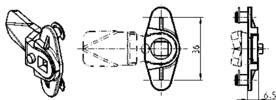
钢锁舌连杆驱动件或不锈钢锁舌连杆驱动件
