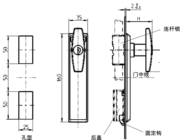
长锁面
